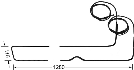
ME1095-3 840W
